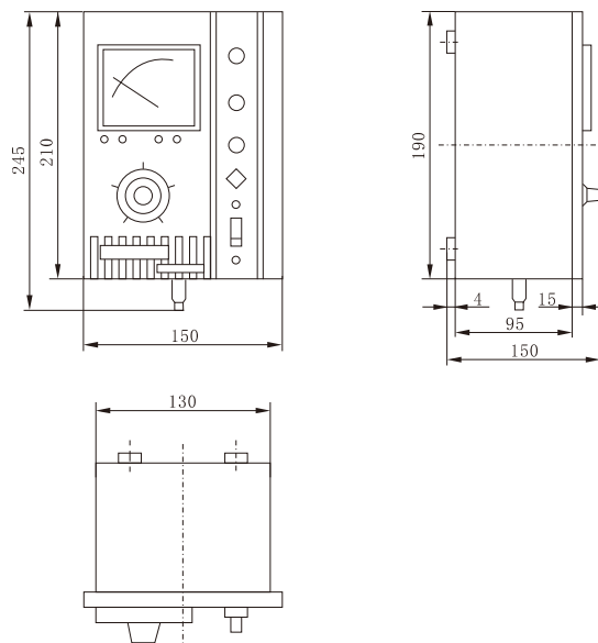
图3 JD1A型外形尺寸
