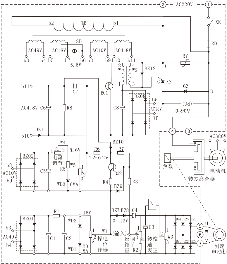
图6 JD1A型电气原理图
