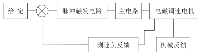
图1 JD1A系列控制装置方框图
