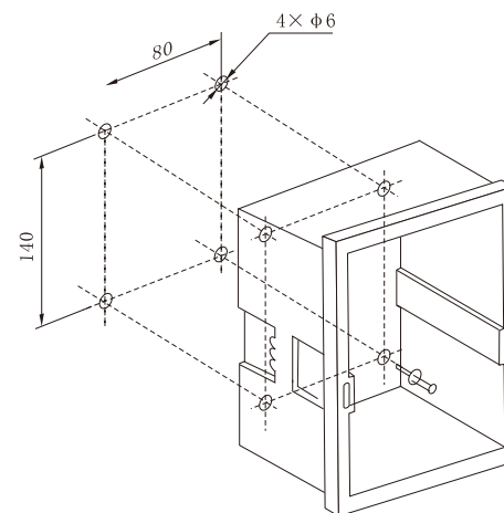
图5 JD1A型用于墙挂式安装尺寸
