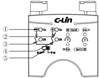
控制面板布局
