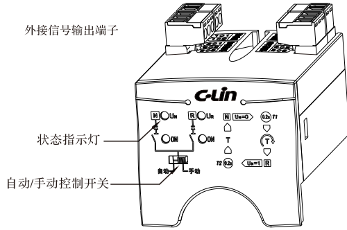
XLNX-A型控制器
