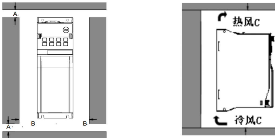
图 4-3 单台安装
