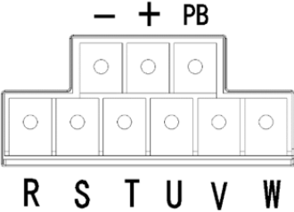
图 4-15 三相 380V 18~37kW 主回路端子（单位：mm）
