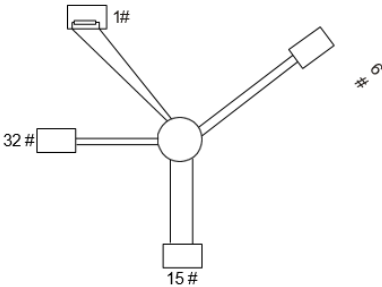
图 10-5 星形接法
