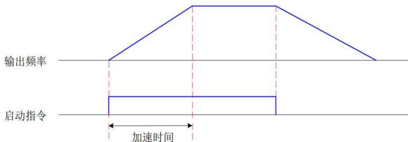
图6-13直接启动时序图
