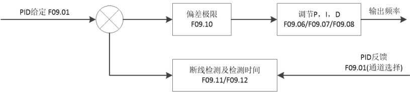
图 6-11 PID控制原理
