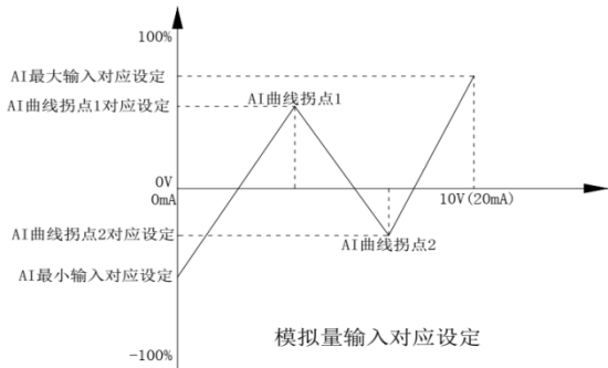
图6-8曲线4和曲线5设定示意图
