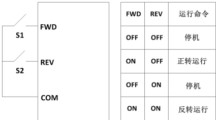
图6-2两线式2
