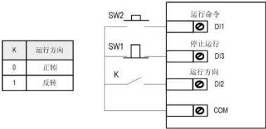
图6-4三线式2
