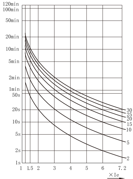
过载保护反时限特性图
